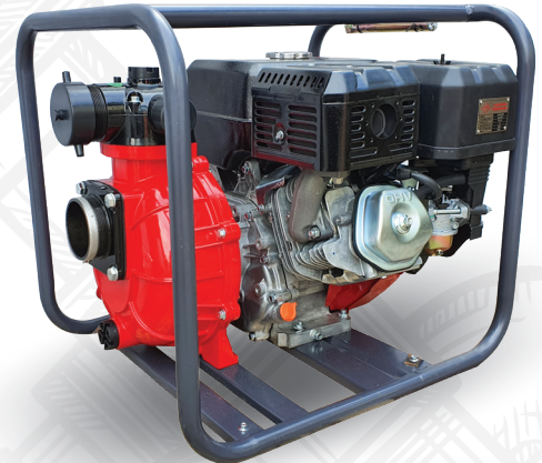
MÁY BƠM XĂNG 15/20HP DI ĐỘNG PORTABLE 15/20HP PETROL PUMP
