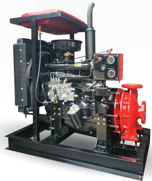
MÁY BƠM DIESEL 4 XI LẠNH 4 CYLINDER DIESEL PUMP
